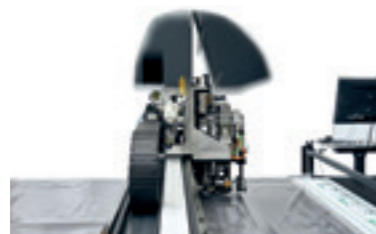
Capot de tête de coupe commandé pneumatiquement avec double mouvement.
