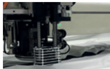
Dispositif de perçage équipé de contrôle de température avec foret ou poinçon.
