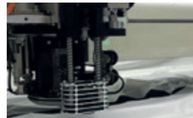
Dispositif de perçage équipé de contrôle de température avec foret ou poinçon.
